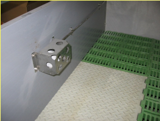
Sensorschutz aus Edelstahl
